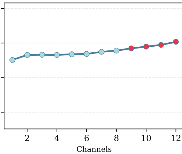
PTB-XL (F1)
