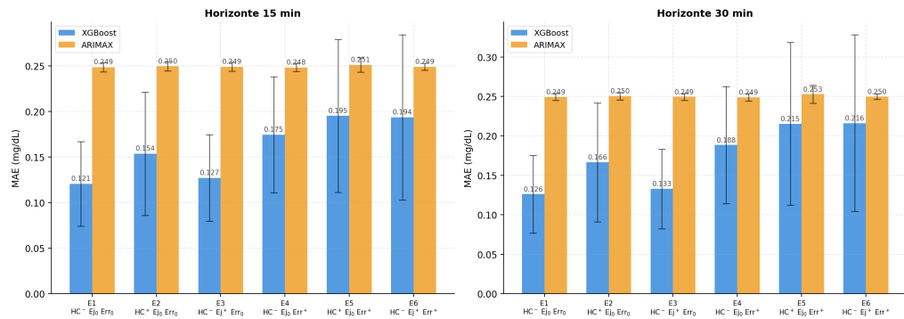
Figura 5.1: Error Absoluto Medio (MAE) promedio por escenario y horizonte de predicción para ARIMAX y XGBoost.
