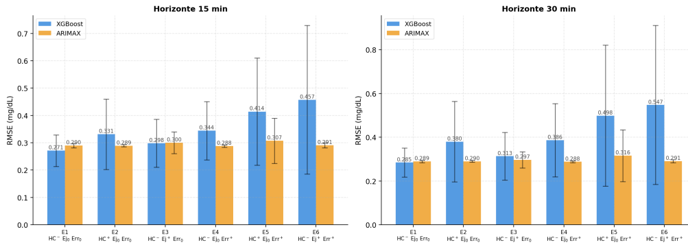
Figura 5.2: Raíz Error Cuadrático Medio (RMSE) promedio por escenario y horizonte de predicción para ARIMAX y XGBoost.
