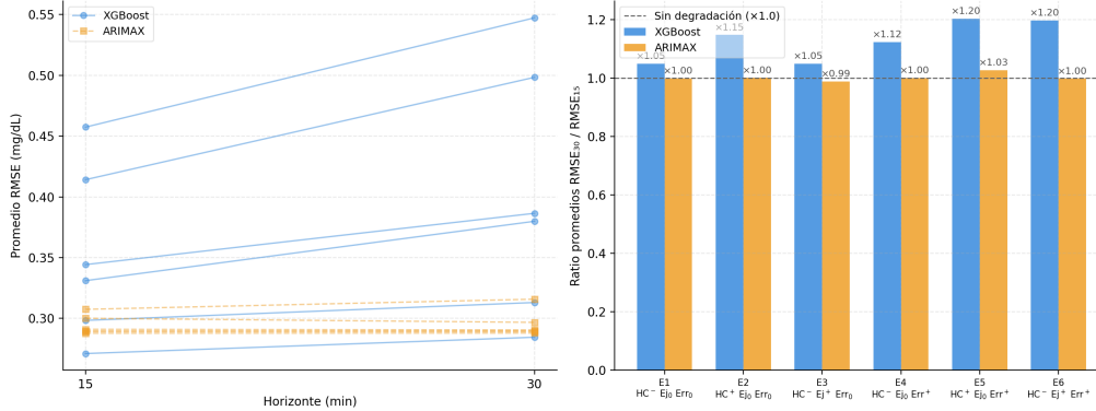
Figura 5.5: Degradación de la Raíz Error Cuadrático Medio (RMSE) al aumentar el horizonte de predicción. Izquierda: valores absolutos por escenario. Derecha: ratio RMSE_{30}/RMSE_{15} por escenario y modelo.
