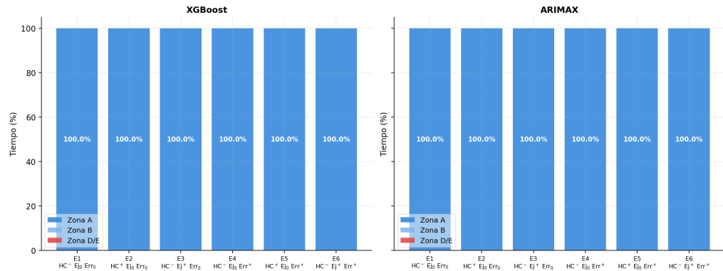
Figura 5.3: Distribución de predicciones en zonas de la Clarke Error Grid (CEG) para XGBoost y ARIMAX en el horizonte de 15 minutos, por escenario.
