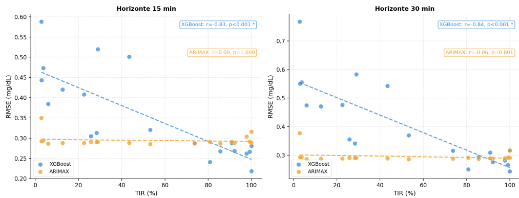
Figura 5.7: Correlación de Spearman entre Raíz Error Cuadrático Medio (RMSE) por paciente (promediado sobre los seis escenarios) y Tiempo en rango (TIR), para ambos modelos y horizontes de predicción.
