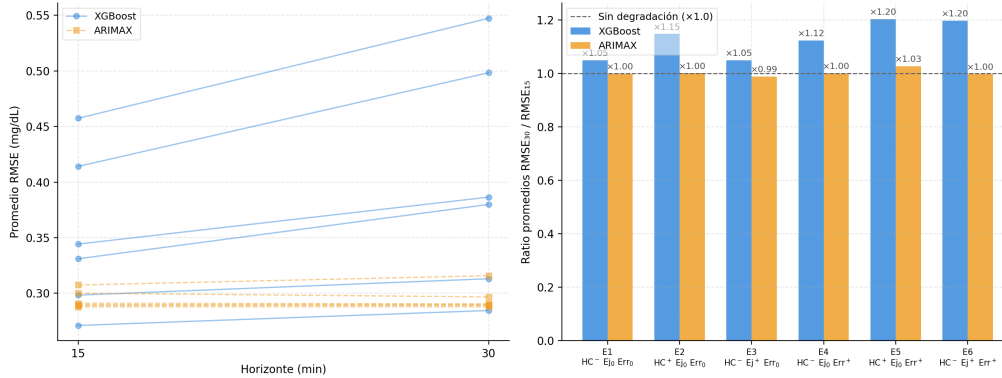
Figura 5.5: Degradación de la Raíz Error Cuadrático Medio (RMSE) al aumentar el horizonte de predicción. Izquierda: valores absolutos por escenario. Derecha: ratio RMSE 30 /RMSE 15 por escenario y modelo.
