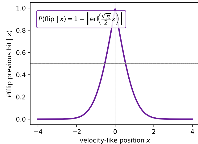
erf V-shaped
