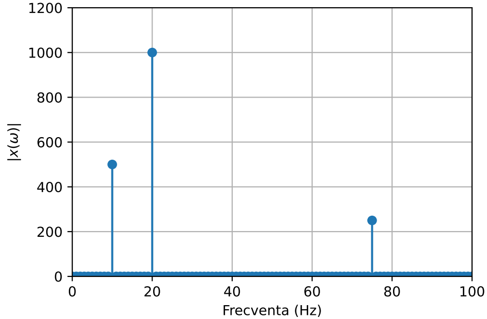
Modulul Transformatei Fourier
