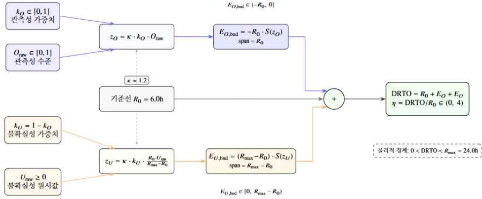
[그림 2-5] DRTO 개별 시그모이드 바운딩 모델 구조
