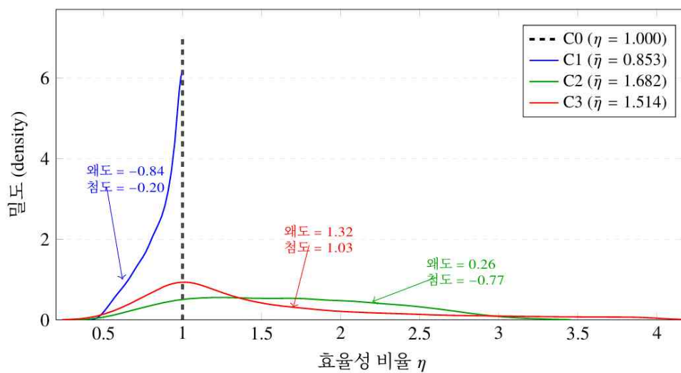
[그림 4-10] C0/C1/C2/C3 효율성 비율 \eta 분포 비교
