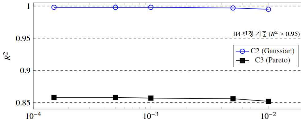
[그림 4-9] LASSO R^2 경로(C2 vs. C3)
