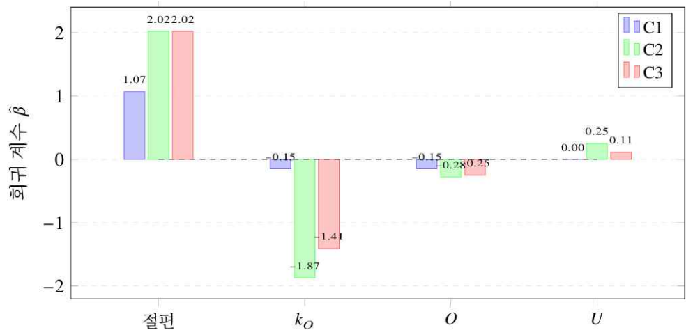
[그림 4-7] C1/C2/C3 1차 다중 회귀 계수 비교
