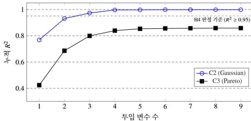
[그림 4-8] 전진 선택법 누적 R^2 진행 비교
