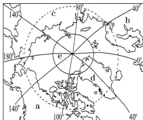
北极地区
