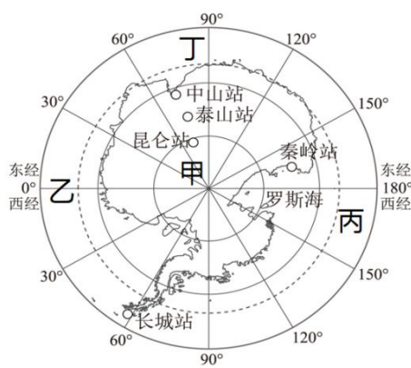
南极地区
