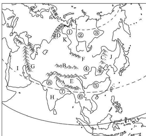
亚洲的地形
