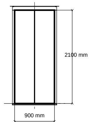
Schachttür · Haltestelle 1 · Vorne
