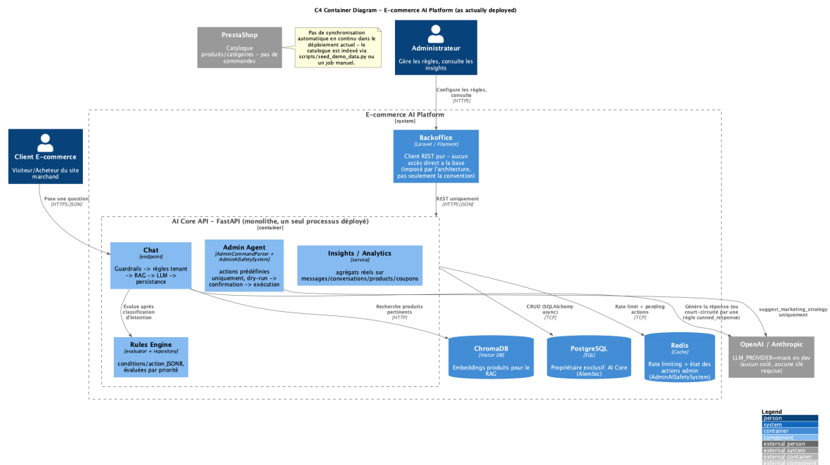
FIGURE 3.1 – Diagramme de conteneurs (C4, niveau 2) de la plateforme
