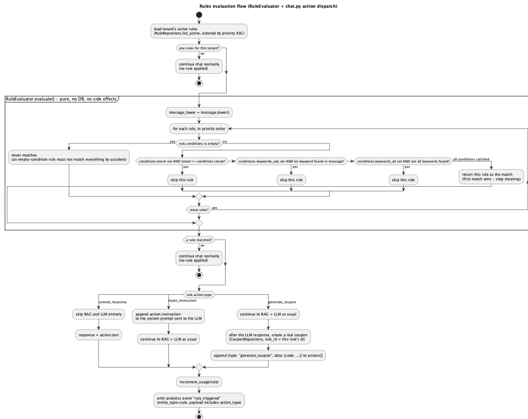
FIGURE 4.1 – Diagramme d’activités : évaluation des règles et répartition des actions
