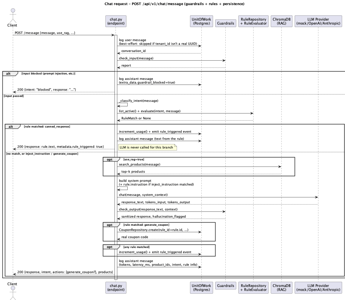
FIGURE 3.4 – Séquence complète d'une requête de chat
