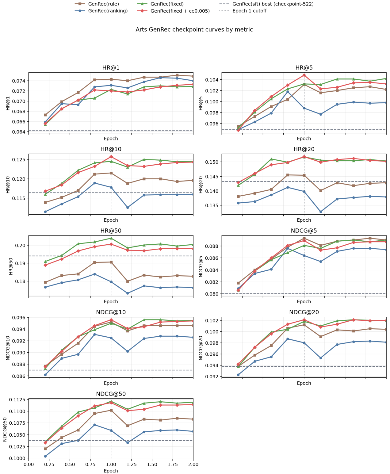
图 9: Arts 上 GenRec RL 变体的完整 checkpoint 曲线。图中统一展示 9 个指标:HR@1/5/10/20/50 与 NDCG@5/10/20/50; 横轴按 Arts RL 主线的 4206 step = 2 epoch 归一化; 虚线表示 GenRec(sft) 的整体 best, 竖向点线表示第一个 epoch 的 cutoff (step \leq 2103)。
