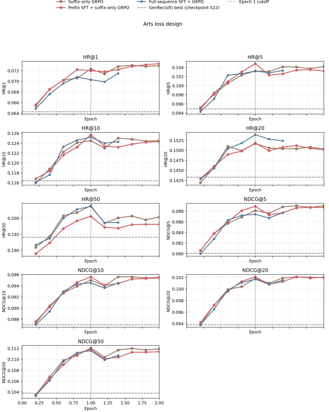
图 4: Arts 上 loss design 对比曲线。图中同时比较 suffix-only GRPO、prefix SFT + suffix-only GRPO 与 full-sequence SFT + GRPO; 横轴按 4206 step = 2 epoch 归一化; 虚线表示 GenRec(sft) 的整体 best, 竖向点线表示第一个 epoch 的 cutoff。如果某条线当前只同步到少量 checkpoint, 则图中会表现为短线或单点。
