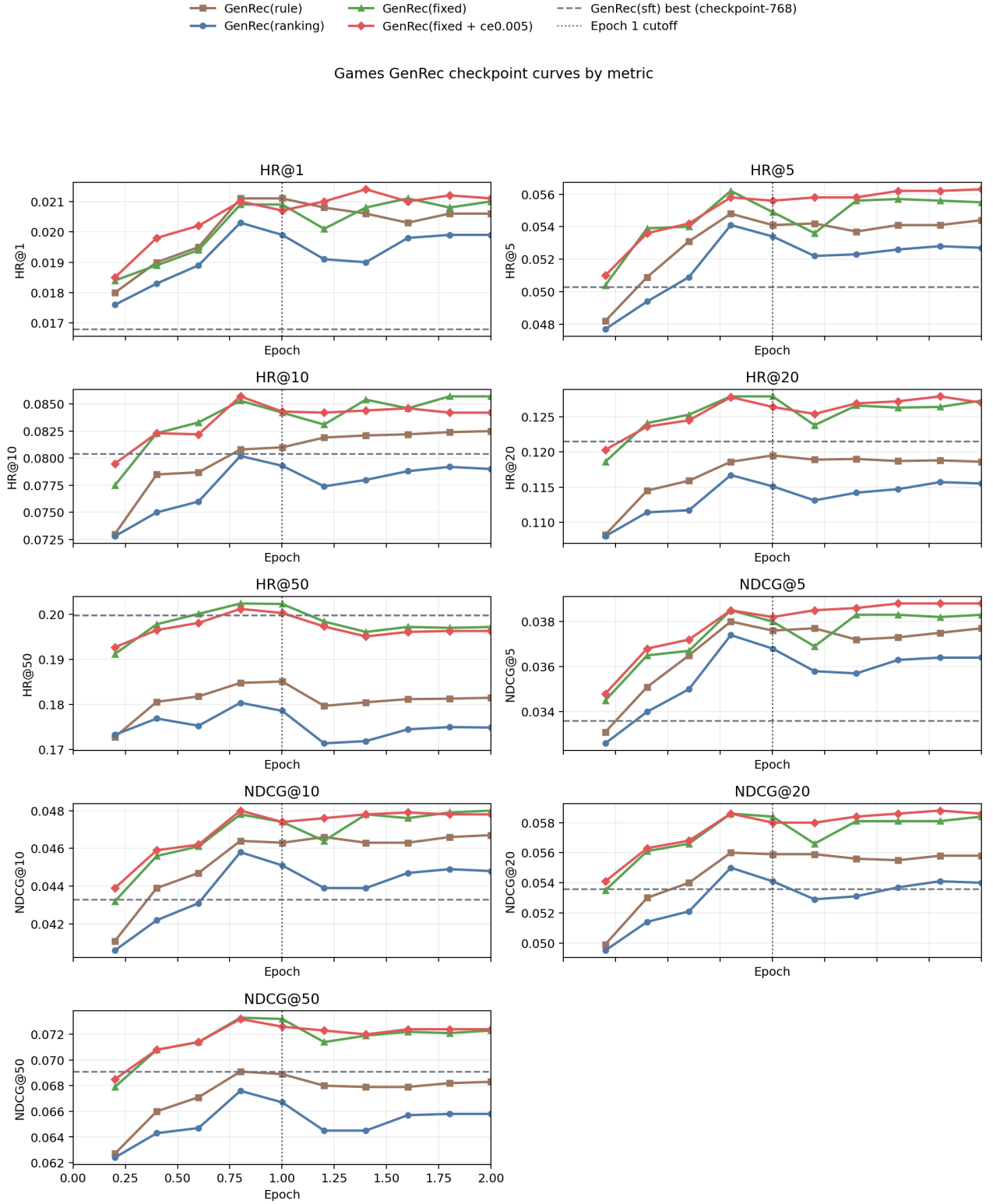
图 8: Games 上 GenRec RL 变体的完整 checkpoint 曲线。图中统一展示 9 个指标: HR@1/5/10/20/50 与 NDCG@5/10/20/50; 横轴按 Games RL 主线的 8752 step = 2 epoch 归一化; 虚线表示 GenRec(sft) 的整体 best, 竖向点线表示第一个 epoch 的 cutoff (step \leq 4376)。
