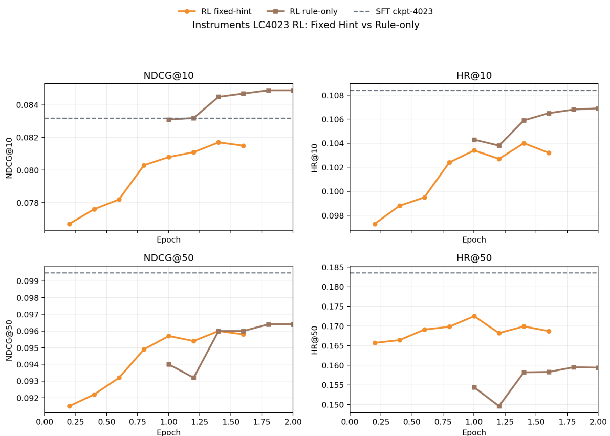
图 1: Instruments 上 lc4023 两条 RL 复现线的 epoch 曲线图。横轴统一按完整训练长度 5006 step = 2 epoch 归一化；fixed-hint 当前只同步到 4008 step，因此曲线在约 1.601 epoch 处结束，虚线表示 SFT ckpt-4023。
