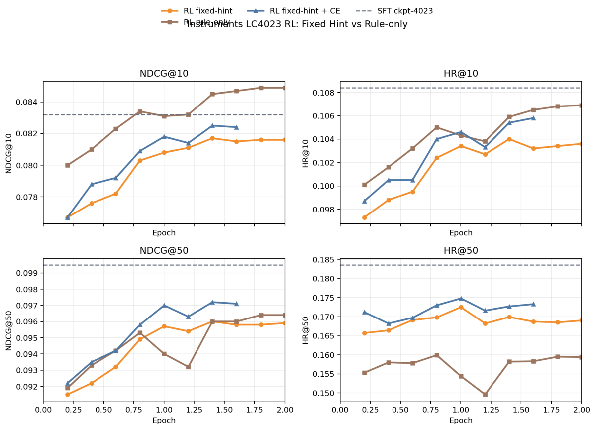
图 2: Instruments 上 lc4023 三条 RL 复现线的 epoch 曲线图。横轴统一按完整训练长度 5006 step = 2 epoch 归一化; fixed 与 rule-only 已同步到 2.0 epoch, fixed-hint + CE 当前同步到约 1.601 epoch, 虚线表示 SFT ckpt-4023。
