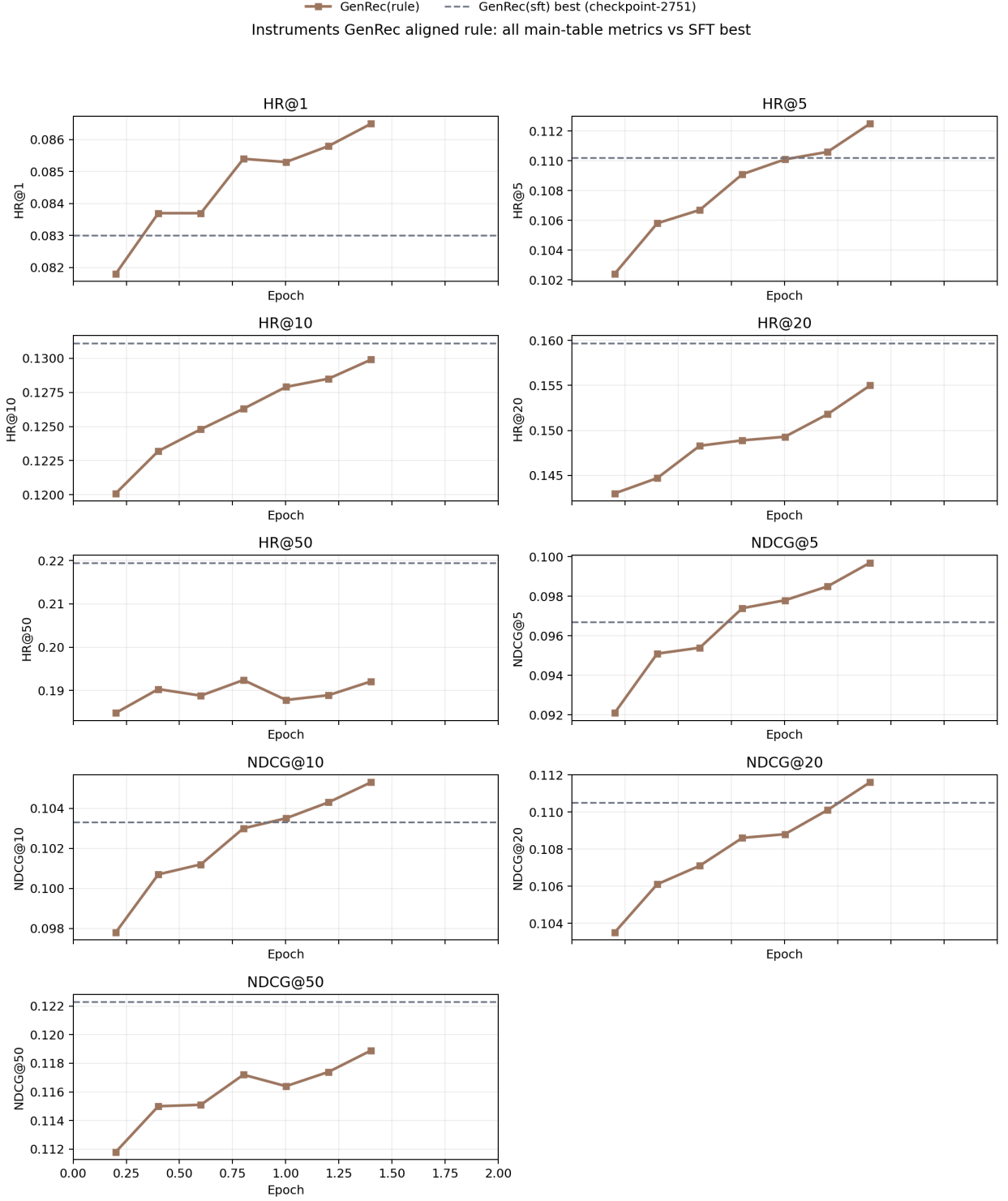
图 1: Instruments 上 GenRec(rule) 的完整 checkpoint 曲线。图中统一展示主表里的九个指标: HR@1/5/10/20/50 与 NDCG@5/10/20/50; 横轴统一按 Instruments RL 主线的 3326 step = 2 epoch 归一化, 因此当前最后一个已同步点 checkpoint-2331 对应约 1.402 epoch, 虚线表示 GenRec(sft)/LC-Rec 共享的最佳 SFT 基线 checkpoint-2751。
