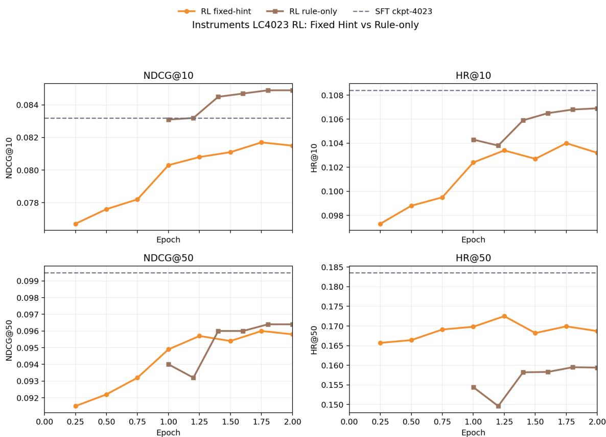
图 1: Instruments 上 lc4023 两条 RL 复现实测的 epoch 曲线图。横轴统一按各自完整训练长度归一化到 2 epoch: fixed-hint 为 4008 step, rule-only 为 5006 step, 虚线表示 SFT ckpt-4023。
