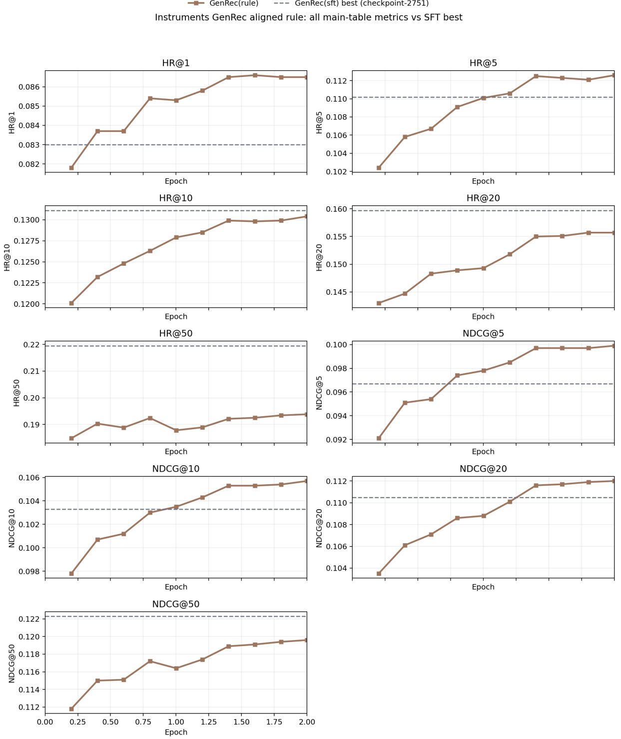
图 1: Instruments 上 GenRec(rule) 的完整 checkpoint 曲线。图中统一展示主表里的九个指标: HR@1/5/10/20/50 与 NDCG@5/10/20/50; 横轴统一按 Instruments RL 主线的 3326 step = 2 epoch 归一化, 因此当前最后一个已同步点 checkpoint-3326 对应约 2.000 epoch, 虚线表示 GenRec(sft)/LC-Rec 共享的最佳 SFT 基线 checkpoint-2751。
