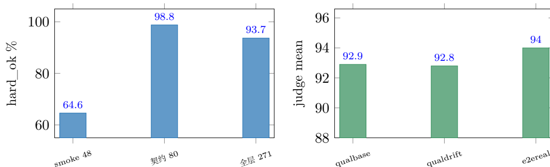
图 7: 翻译侧演化。左: swe-2-medium 硬契约率——09-15 smoke 期网关不稳（http_err 17）压到 64.6%，契约批 98.8%，今日全层抽样 93.7%（新校验口径 v_err 27 条计入后更严）；右: ESA judge 均分 92.9→94.0（swe-2-max 评审，contested 8.1%→5.5% 下降）。
