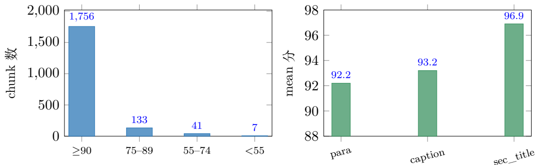
图 10: qualbench 评分分布 (左: 分数段; 右: per-kind 均分)。1,756/1,937 chunk \geq 90 ; para 类是主要拉低项 (flag 榜: term_inconsistency 229、grammar 197、mistranslation 132、hallucinated_content 66)。
