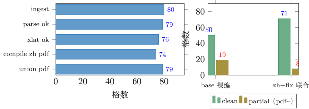
图 9: stagerun 五阶段漏斗与同格对照 (80 篇跨层样本, xlat 为 mock 上游)。左: 主流水线 zh 臂逐段存活数; 右: 同一 80 格上 base 裸编译 vs zh+fixloop union 终态——管线相对裸编译 pdf +10 格、clean +21 格 (fixloop 救回 fail 5 格全升 clean、partial 5 格升 clean)。
