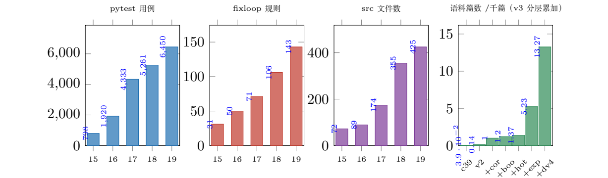
图 8: 资产增长 (git 历史抽样, 同日口径一致): pytest 798→6,450、fixloop 规则 31→143 (16 分片)、src 72→425 文件、语料 corpus39/v2 → v3 八层 13,266 (另有 corpus_daily 日更渠 ~1,200 篇/日在库外增长)。
