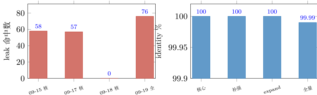
图 6: 解析侧演化。左: leak 命中数——dollar 族 58/57 条残留于 09-18 c2-dollar 车道清零（核心层口径），09-19 全量 28,904 文件上重现 76 条（1,845,338 chunk 中 0.004%，新语料表面新案例，非回归）。右: strict identity 全测量期 \geq 99.99\% （纵轴截断）。
