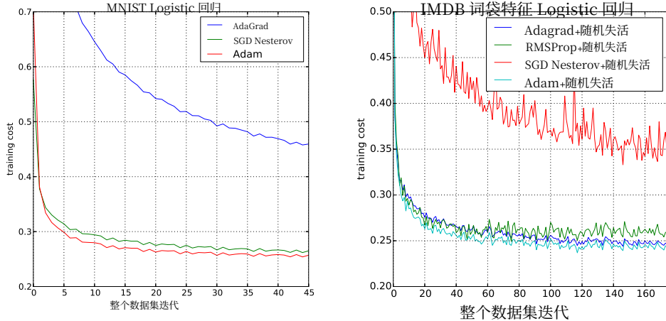
图 1: 在 MNIST 图像和带有 10,000 维词袋 (BoW) 特征向量的 IMDB 电影评论上, Logistic 回归训练的负对数似然。
