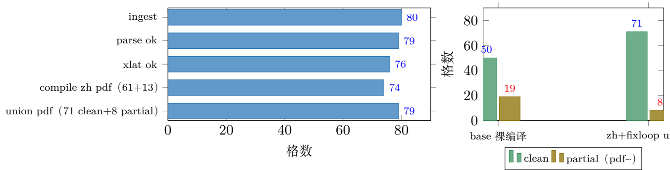
图 8: stagerun 五阶段漏斗与同格对照 (80 篇跨层样本, xlat 为 mock 上游)。左: 主流管线 zh 臂逐段存活数; 右: 同一 80 格上 base 裸编译 vs zh+fixloop union 终态——管线相对裸编译 pdf +10 格、clean +21 格 (fixloop 救回 fail 5 格全升 clean、partial 5 格升 clean)。
