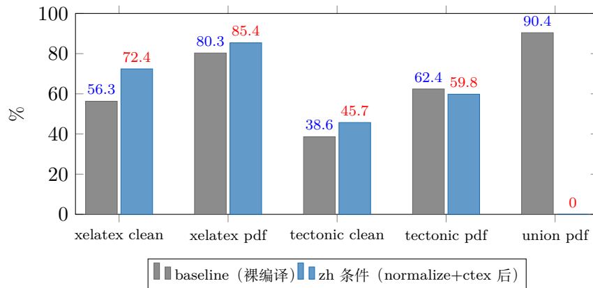
图 10: compilebench 500 格: baseline vs zh 条件。zh 臂 xelatex clean +16.1pt——normalize 修复了源级缺陷; union pdf 90.4% (双引擎取优)。
