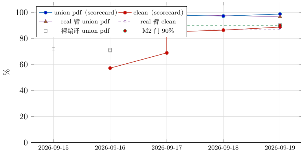
图 4: 编译健康度时间线。scorecard 线为 stagerun records 在代码演进下的重评 (loop1 n=5124 \rightarrow loop2 n=5219 \rightarrow v3all 样本 n=80 )；real 臂为真 LLM 翻译全链 (realn200 \rightarrow e2e-v3b n=60 终态)；方块为裸编译基线——注意基线自身四天涨 \sim 19\text{pt} (71.7 \rightarrow 90.2)：vendored 宏包资产 + tlmgr usertree 积累使工具链整体成熟，「裸引擎撑死七成」的 09-15 结论已不适用今日地板。
