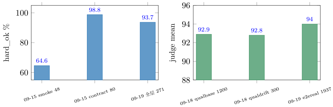
图 6: 翻译侧演化。左: swe-2-medium 硬契约率——09-15 smoke 期网关不稳 (http_err 17) 压到 64.6%, 契约批 98.8%, 今日全层抽样 93.7% (新校验口径 v_err 27 条计入后更严); 右: ESA judge 均分 92.9→94.0 (swe-2-max 评审, contested 8.1%→5.5% 下降)。
