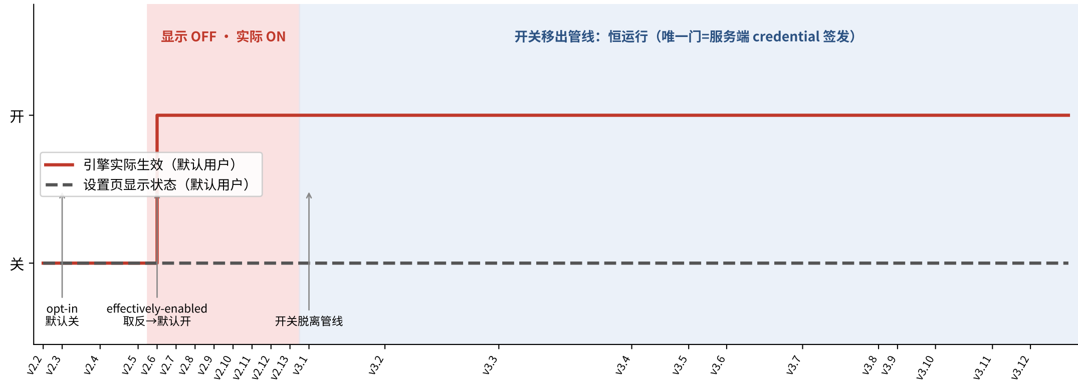
同意门三阶段：界面显示与引擎生效的背离（默认配置、未手动改动开关的用户）
