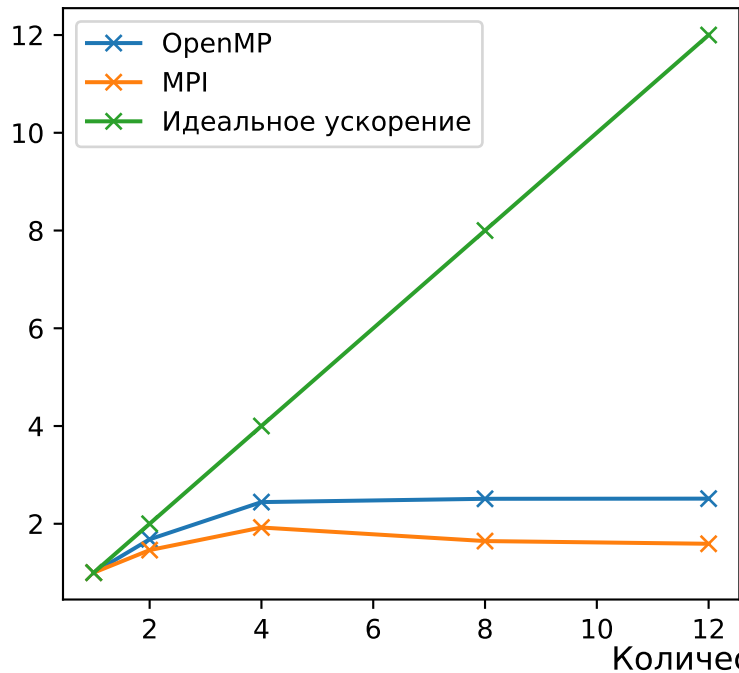
Ускорение в зависимости от количества потоков, раз
