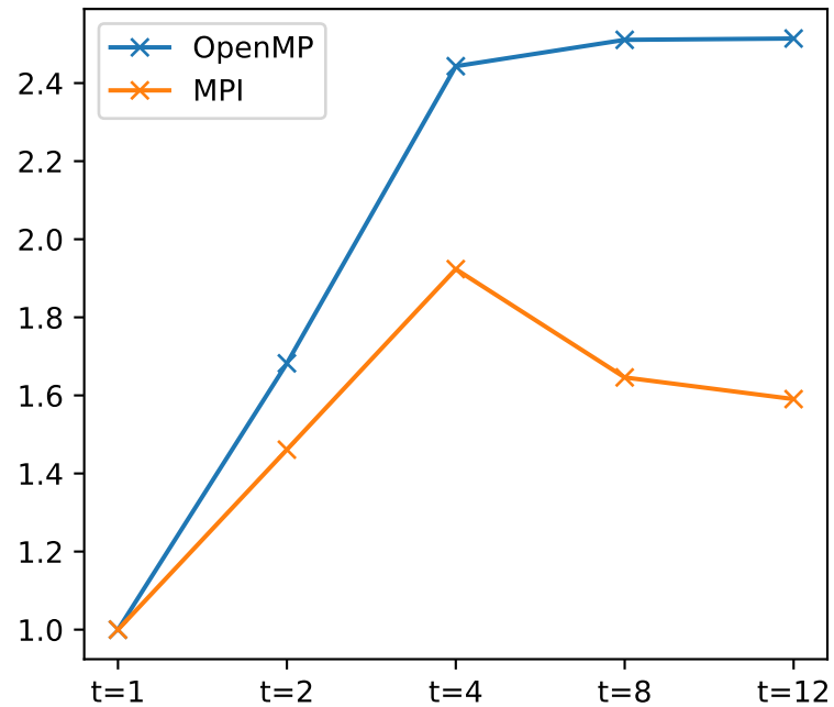
Ускорение в зависимости от количества потоков, раз
