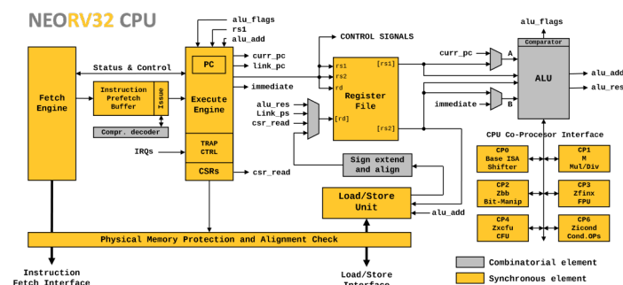
Abbildung 5.1: NEORV32 Architektur
