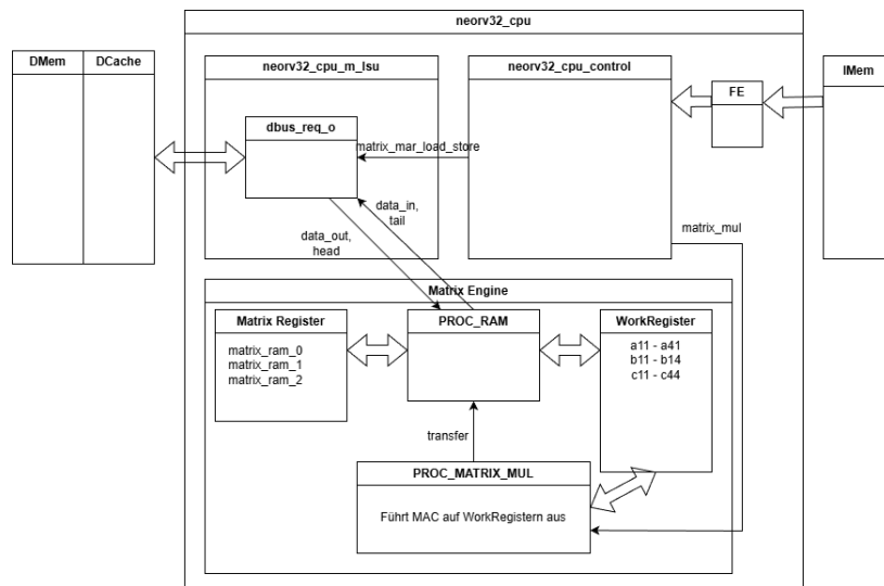
Abbildung 5.1: VHDL Entities
