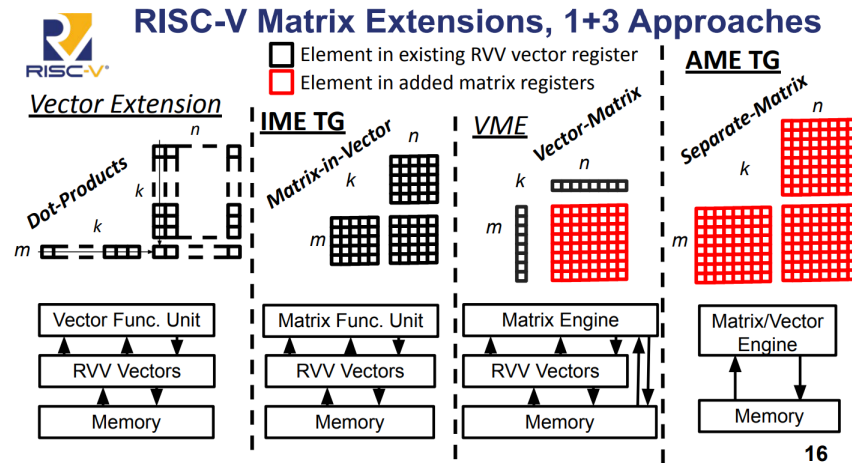
Abbildung 2.3: Ansätze zur Matrix-Extension
