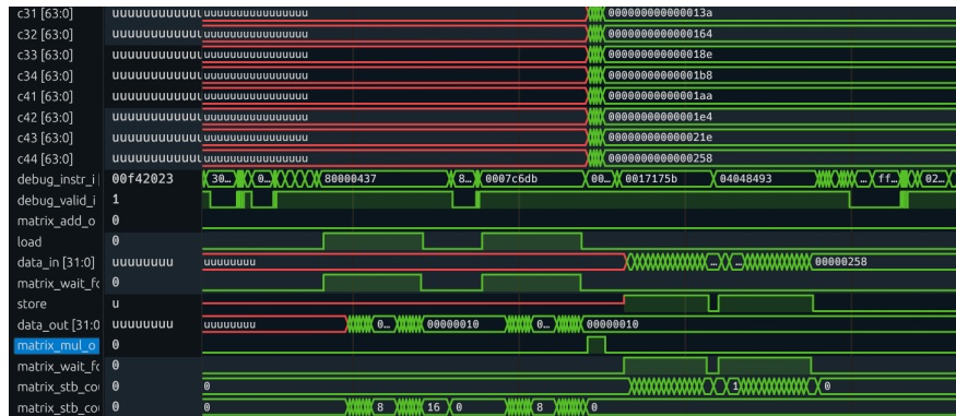
Abbildung 6.1: Steuersignale der Matrixmultiplikation
