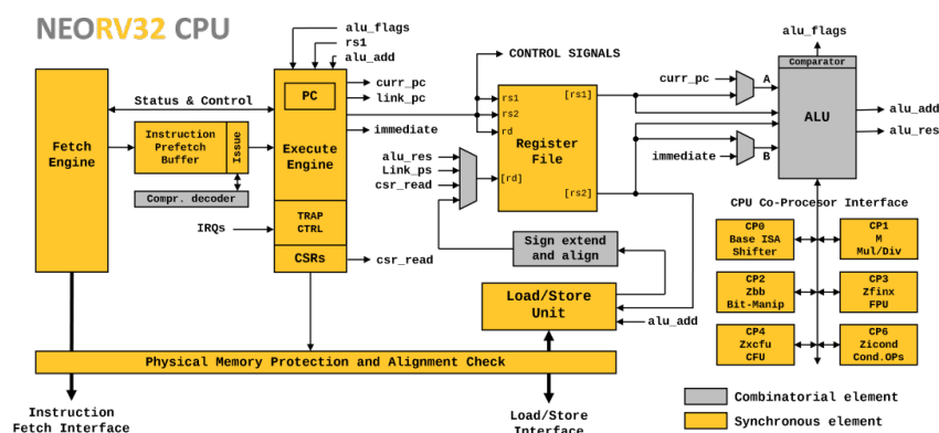
Abbildung 4.1: NEORV32 Architektur
