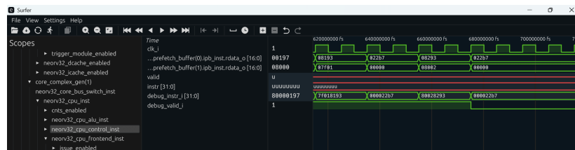
Abbildung 5.2: NEORV32 Gültige Instruktion
