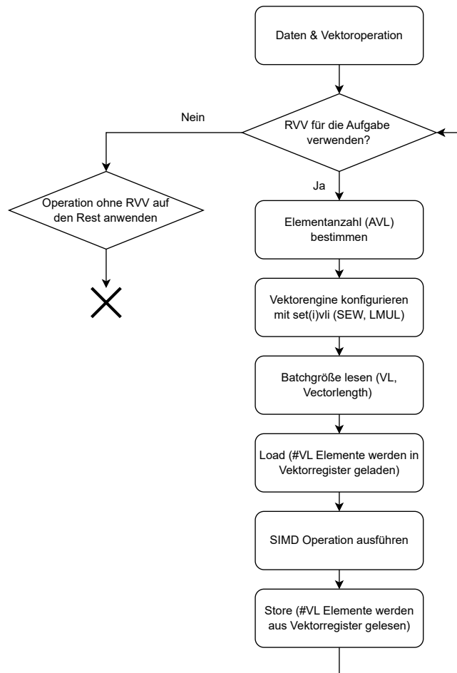
Abbildung 2.3: Strip-Mining Ablauf
