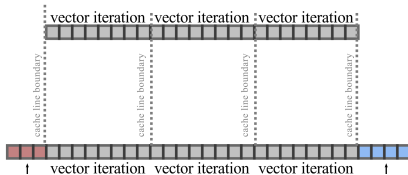
Abbildung 1.5: Strip Mining (Quelle: [19])
