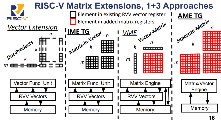
Abbildung 2.4: Ansätze zur Matrix-Extension (Quelle: [4], S.16)
