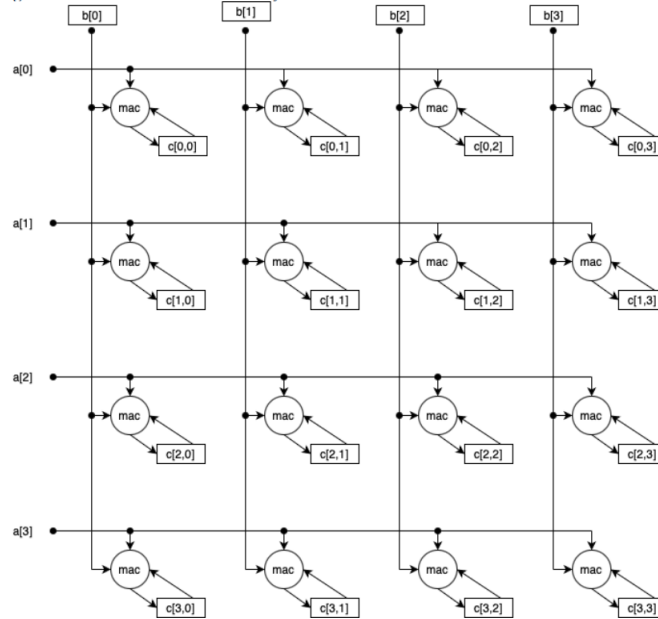
Abbildung 2.10: Matrix Accumulator (MAC) (Quelle: [11], S.23)
