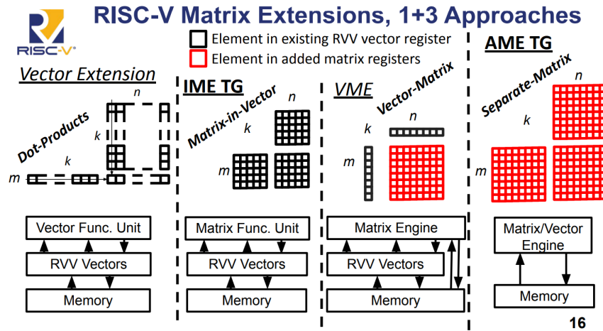
Abbildung 2.1: Ansätze zur Matrix-Extension
