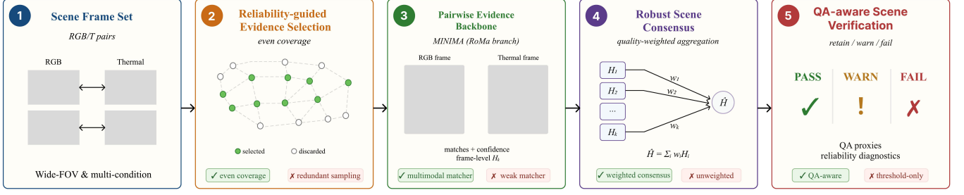
图 2: UAV-TAlign 参考框架。渐进式证据调度从 MINIMA-RoMa 骨干获得逐帧单应性；几何校准权重、中位数/MAD 共识和跨模态验证进一步将逐帧假设转化为规范场景产品。
