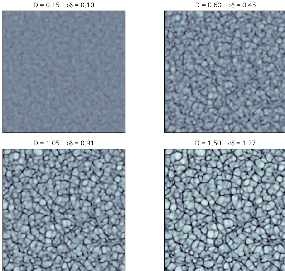
그림 4 채택한 Zel'dovich 규칙에서 성장하는 뒤틀림 응력의 밀도 표현형
