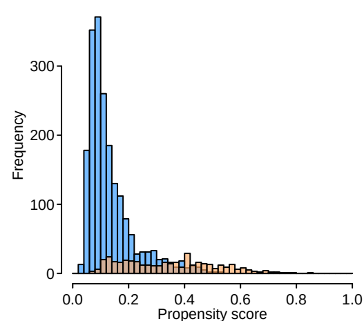
Estimator: GBM
