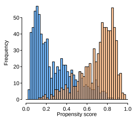
Estimator: GBM
