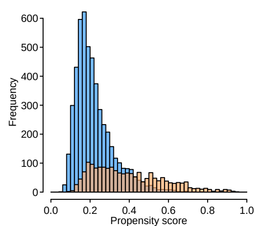
Estimator: GBM
