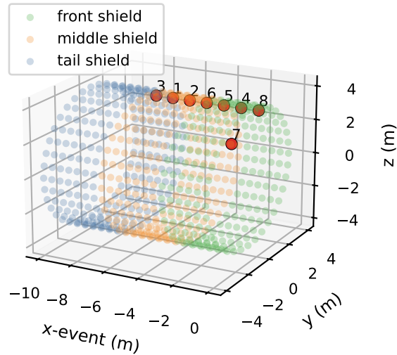
A. Local 3D rock-shield edge provenance
