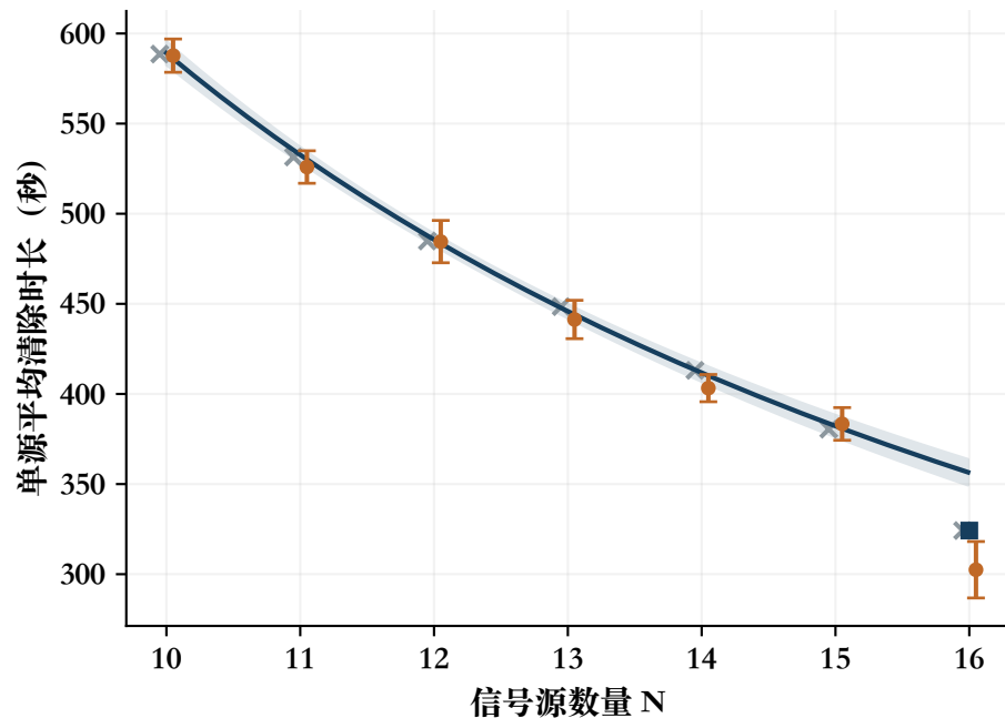
Q4: 全向与定向混合
