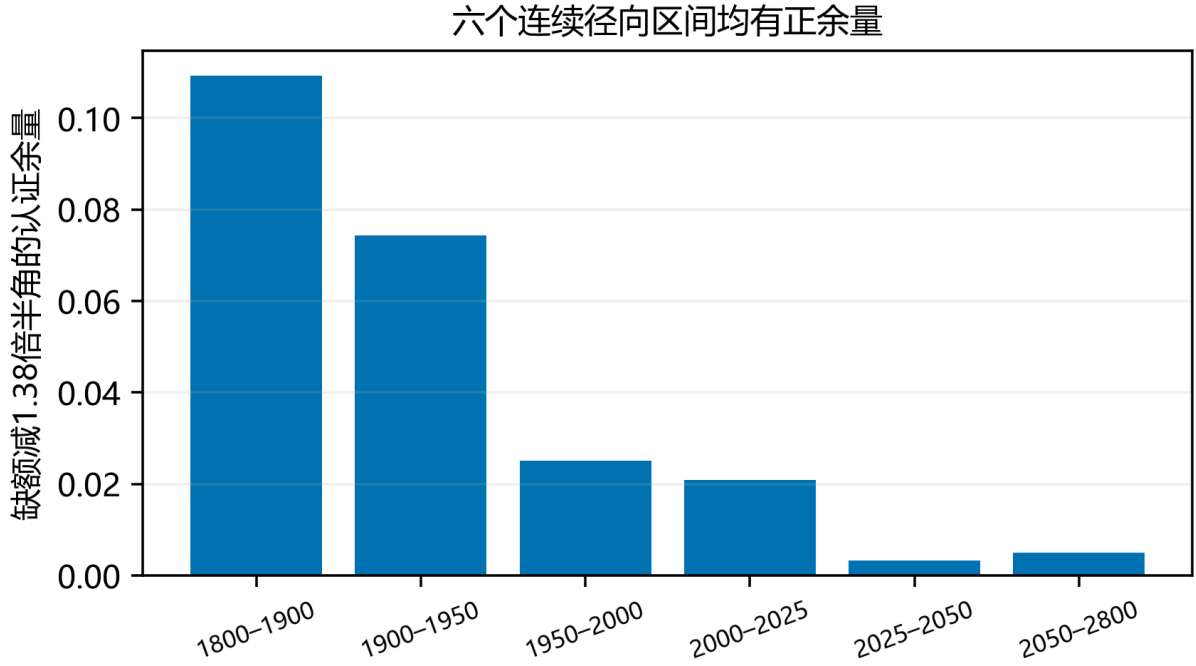
图 1: 面积缺额与边界弧的六个连续区间证书, 显示的余量均为正。
