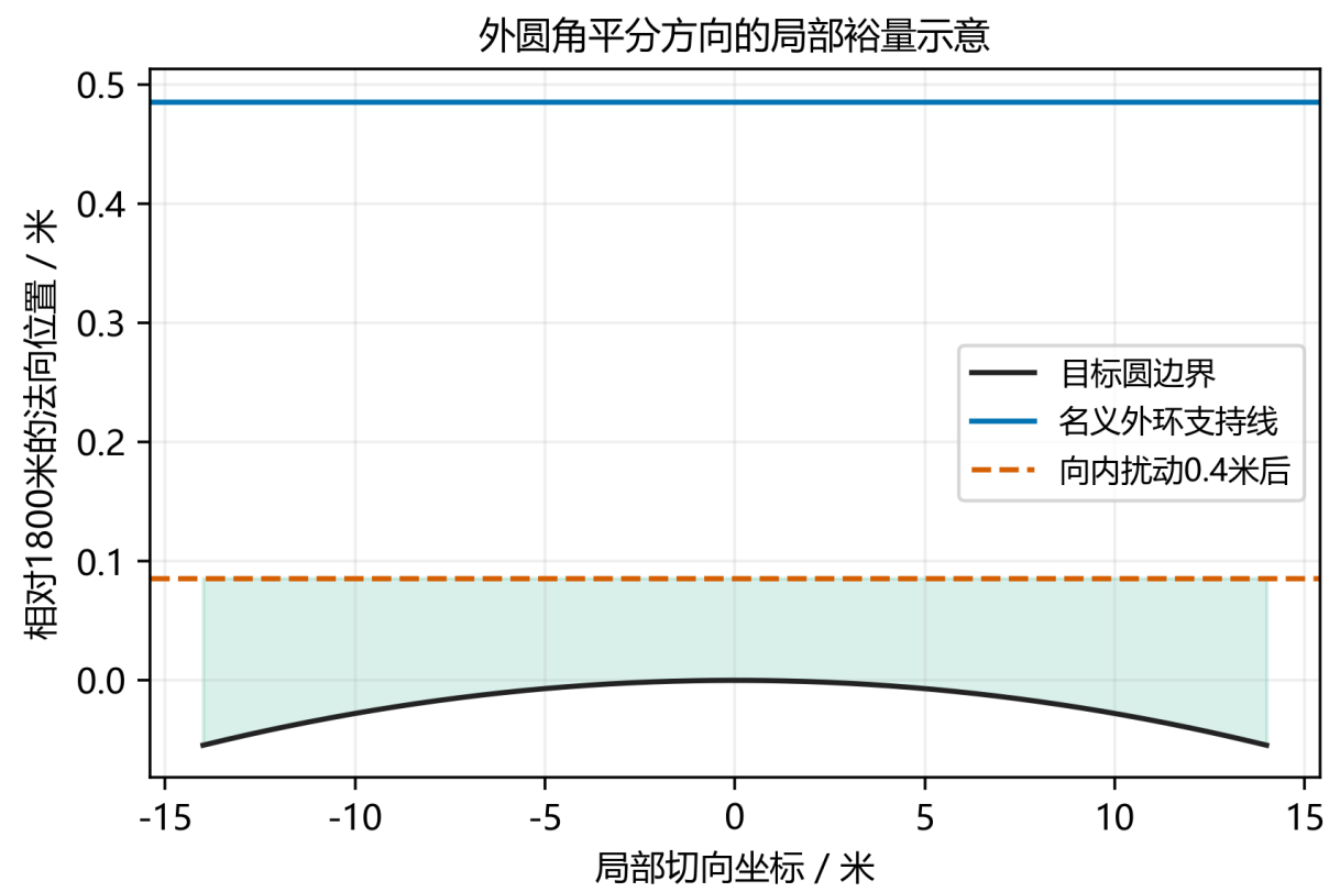
图 2: 外圈角平分方向的局部放大示意。整圆与所有方向的结论由连续证书给出，图仅解释一个限制方向。
