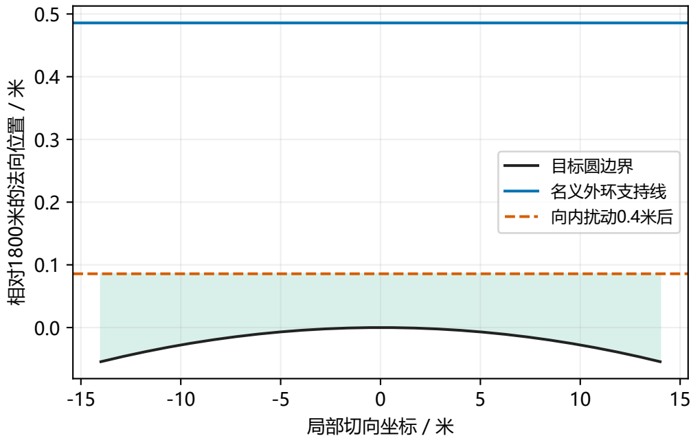
外圆角平分方向的局部裕量示意
