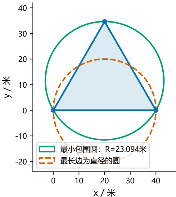
(a) 直径与覆盖圆反例
