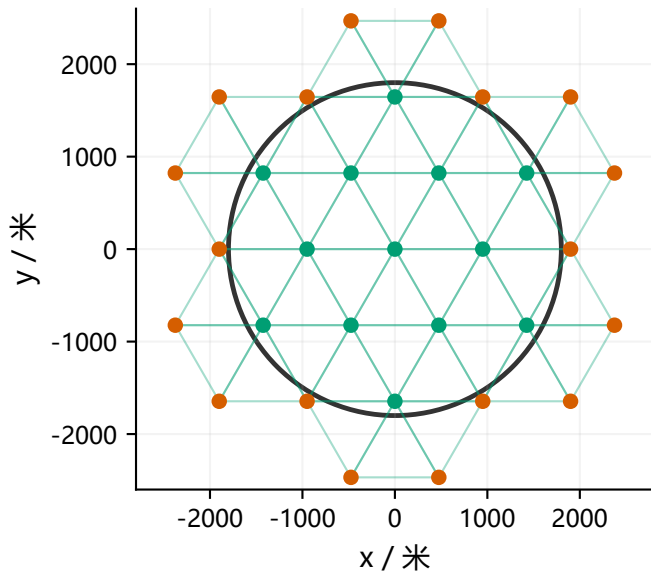
(b) 定向31点：三角格边长950米
