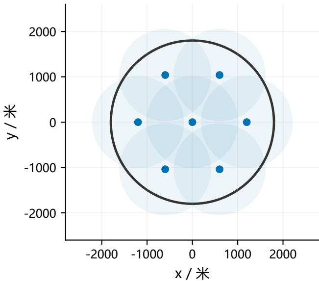
(a) 全向7点：覆盖半径968.902米
