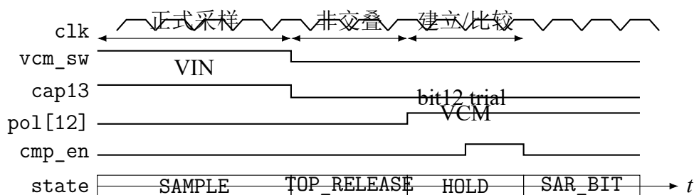
图 10-3 正式采样、保持与 MSB trial 时序图
