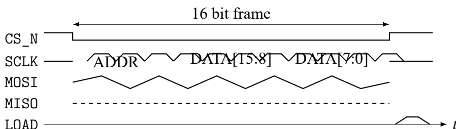
图 10-2 SPI 寄存器配置协议时序图
