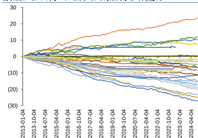
图表22: GPT 因子工厂 2.0 产出的高频因子累计周度 IC
