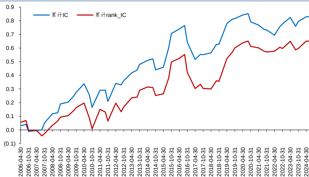
图表14：GPT 因子工厂 2.0 产出的基本面因子实例累计周度 IC 和 RankIC
