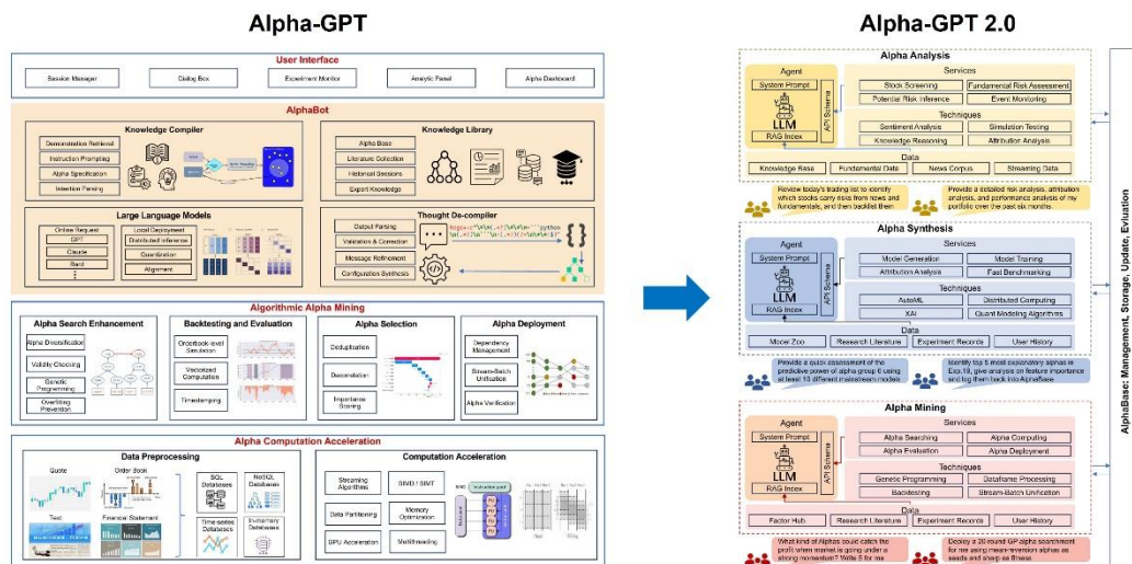
图4：Alpha-GPT 与 Alpha-GPT 2.0 因子挖掘框架
