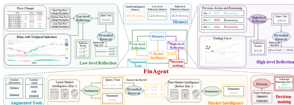
图表2：FinAgent 架构
