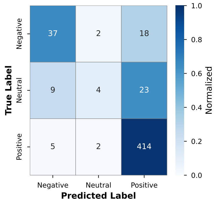
SVM
