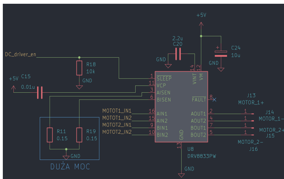
Rysunek 2.10: Schemat elektryczny mostka H.
