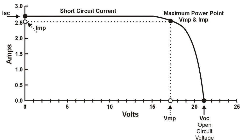
Rysunek 2.2: Wykres prądu w funkcji napięcia panelu.
