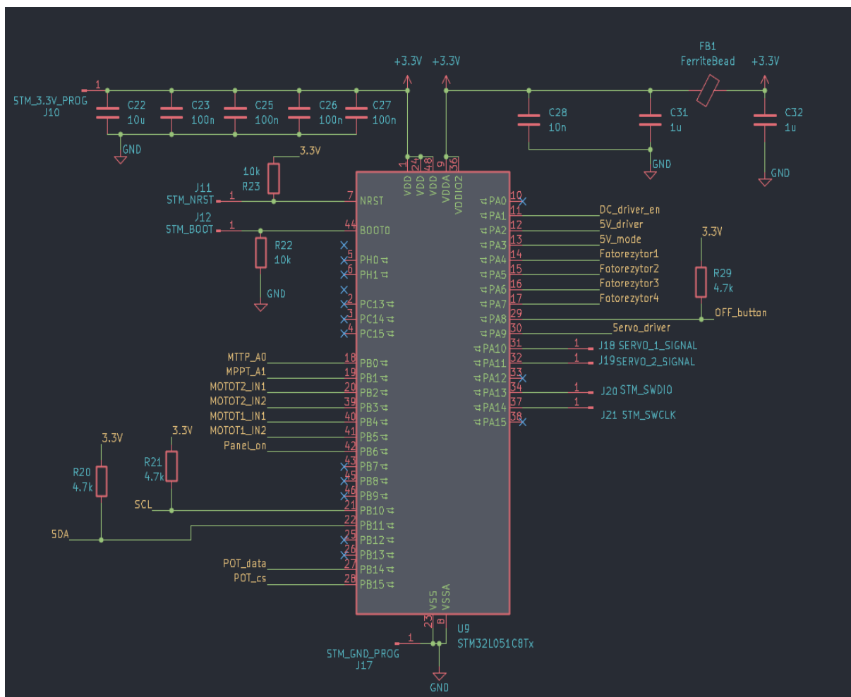
Rysunek 2.6: Schemat elektryczny mikrokontrolera.
