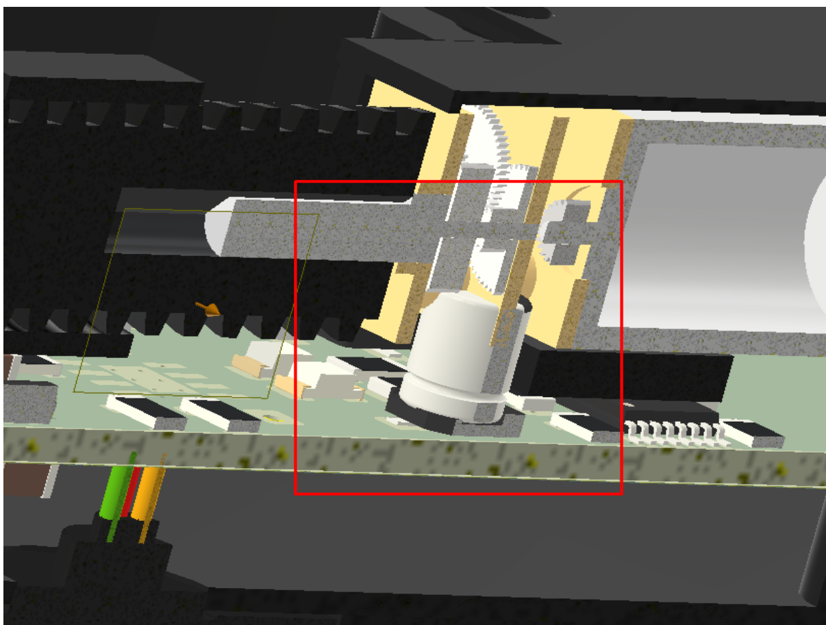
Rysunek 5.2: Przekrój modelu urządzenia pokazujący położenie płytki PCB, silnika oraz elementów mechanicznych.
