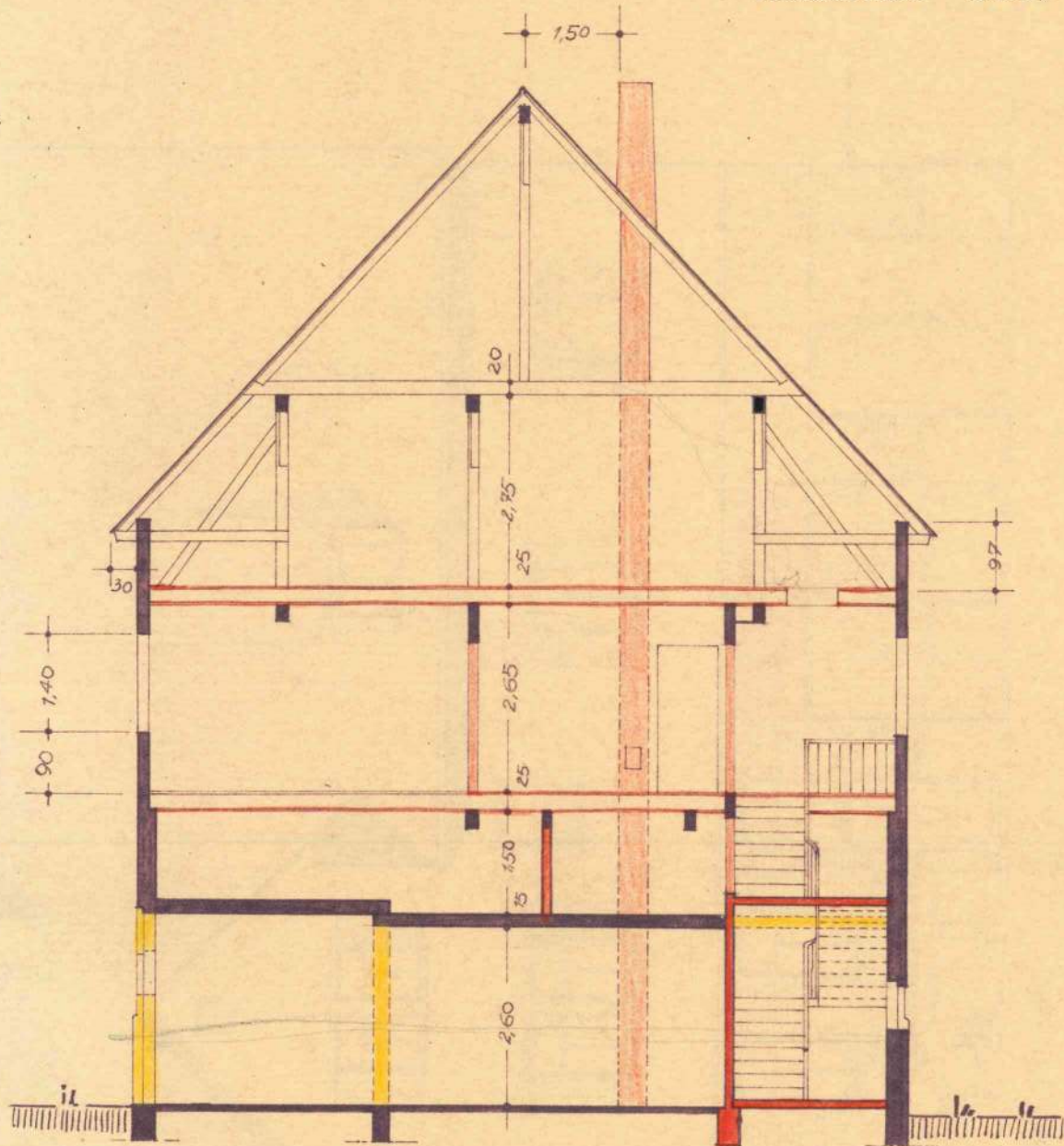
Querschnitt
