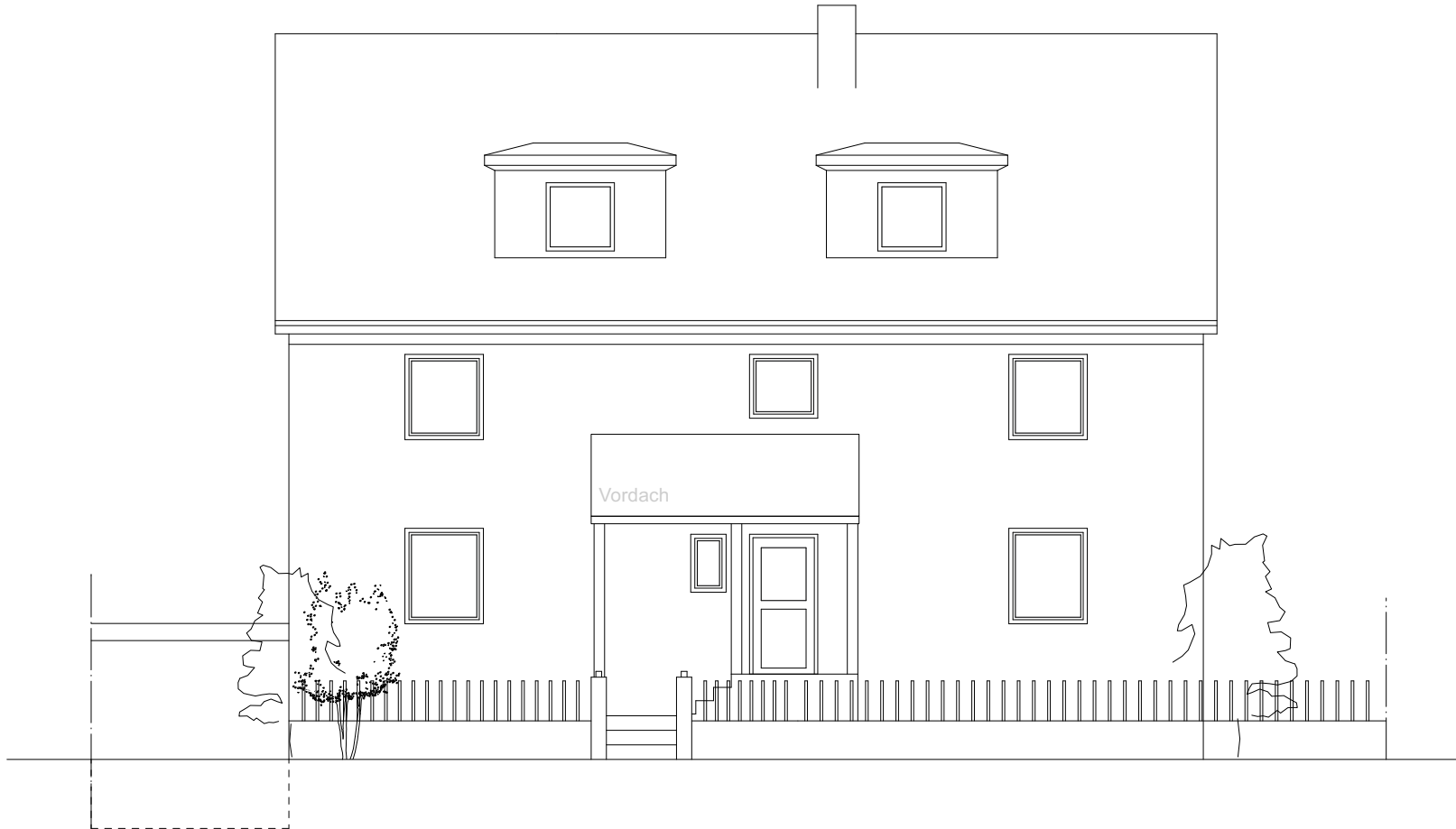
Ansicht Nordseite
