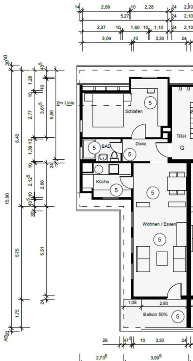
Abbildung 10: Grundriss Wohnung Nr. 5
