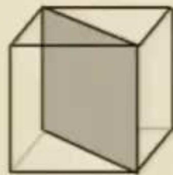
(110)
