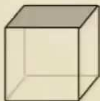
(001)
