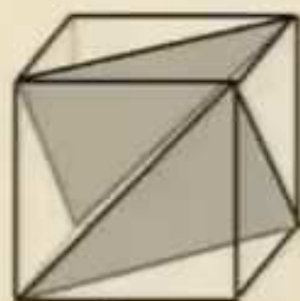
(\bar{1}11)
