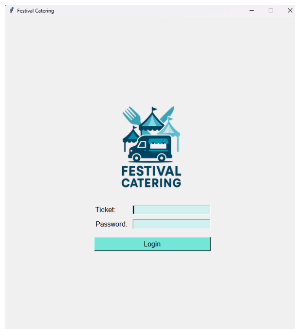
Abbildung 11: Login-Seite
