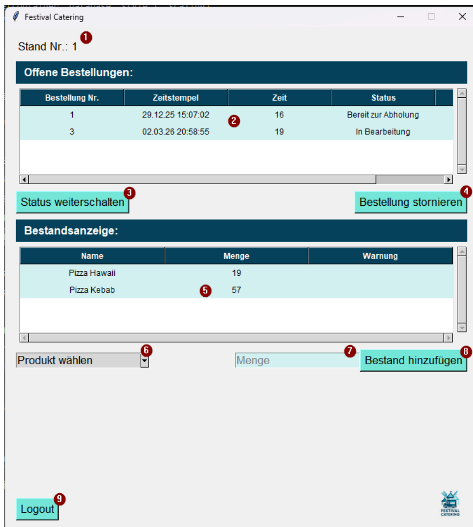
Abbildung 14: Verkäufer-Seite
