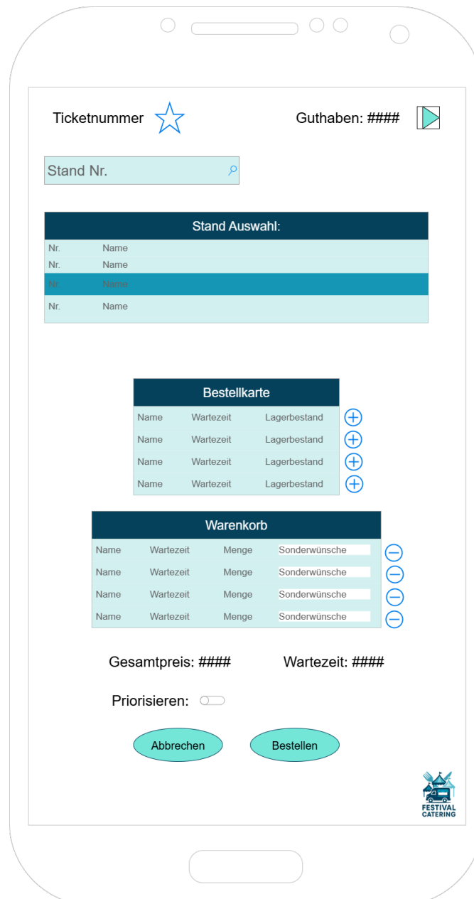
Abbildung 4: Mockup: Bestells-Seite
