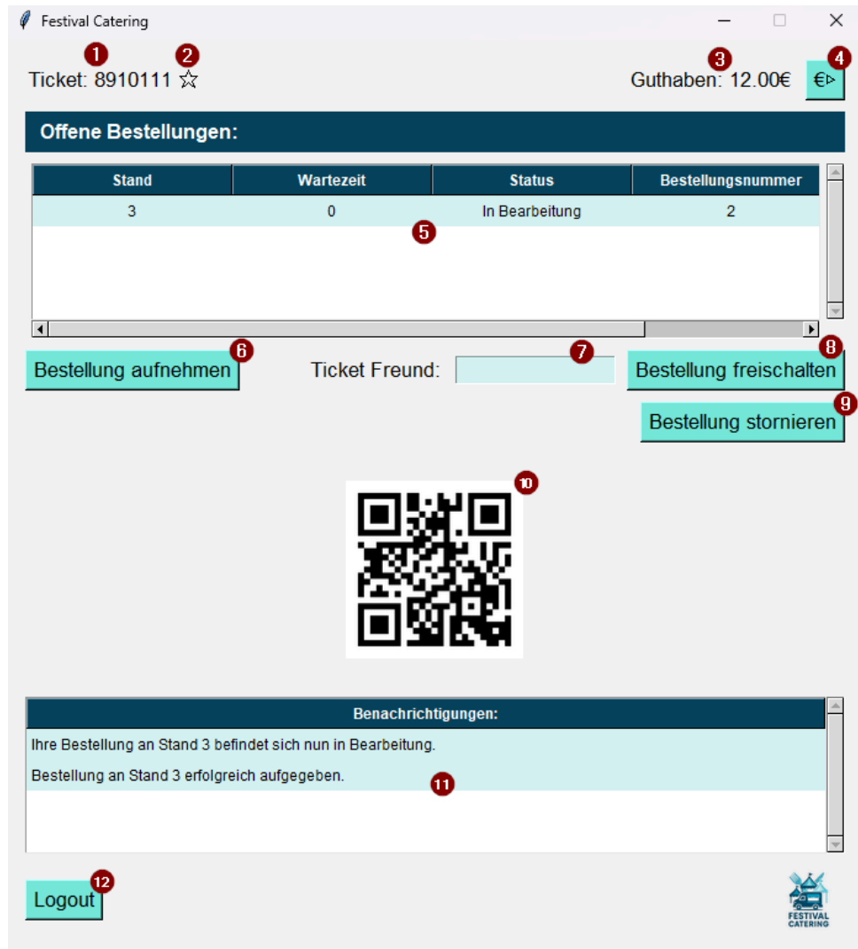
Abbildung 12: Besucher-Seite
