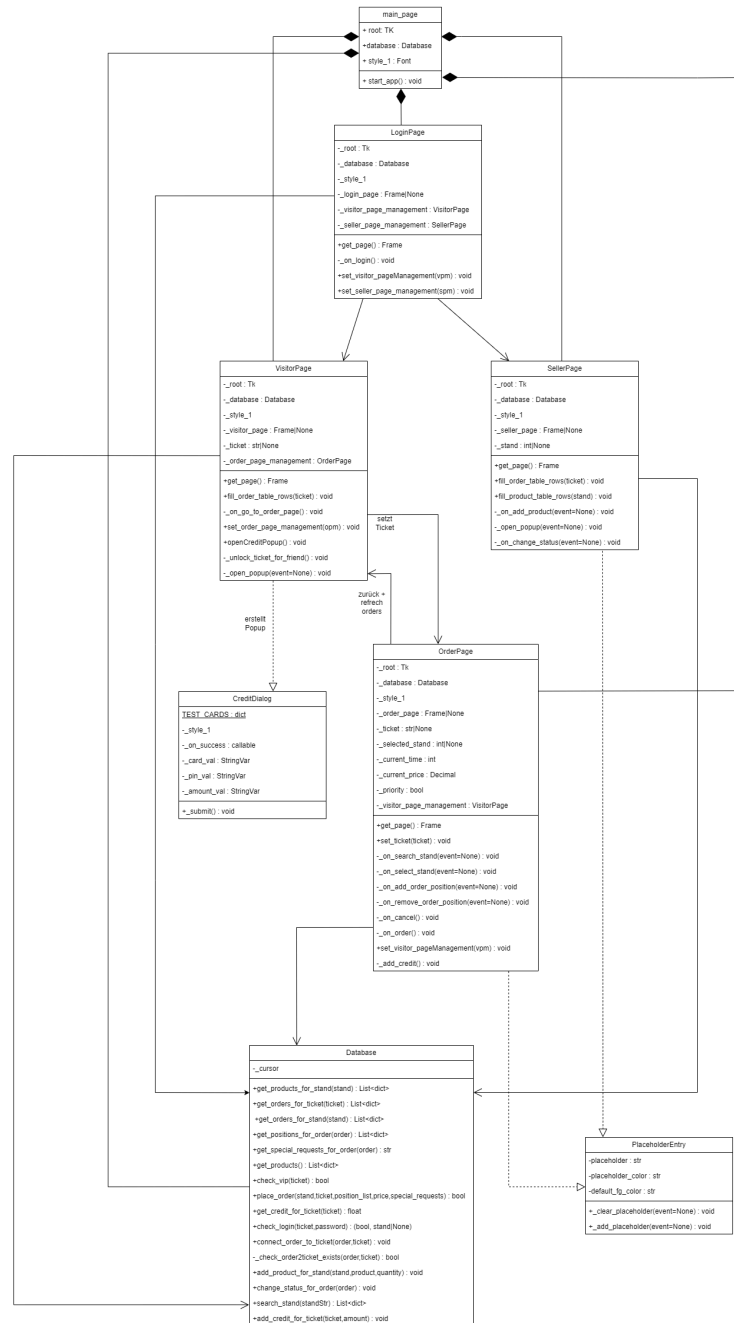
Abbildung 10: Klassendiagramm
