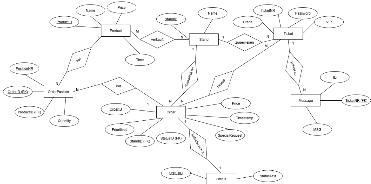
Abbildung 8: ER-Diagramm
