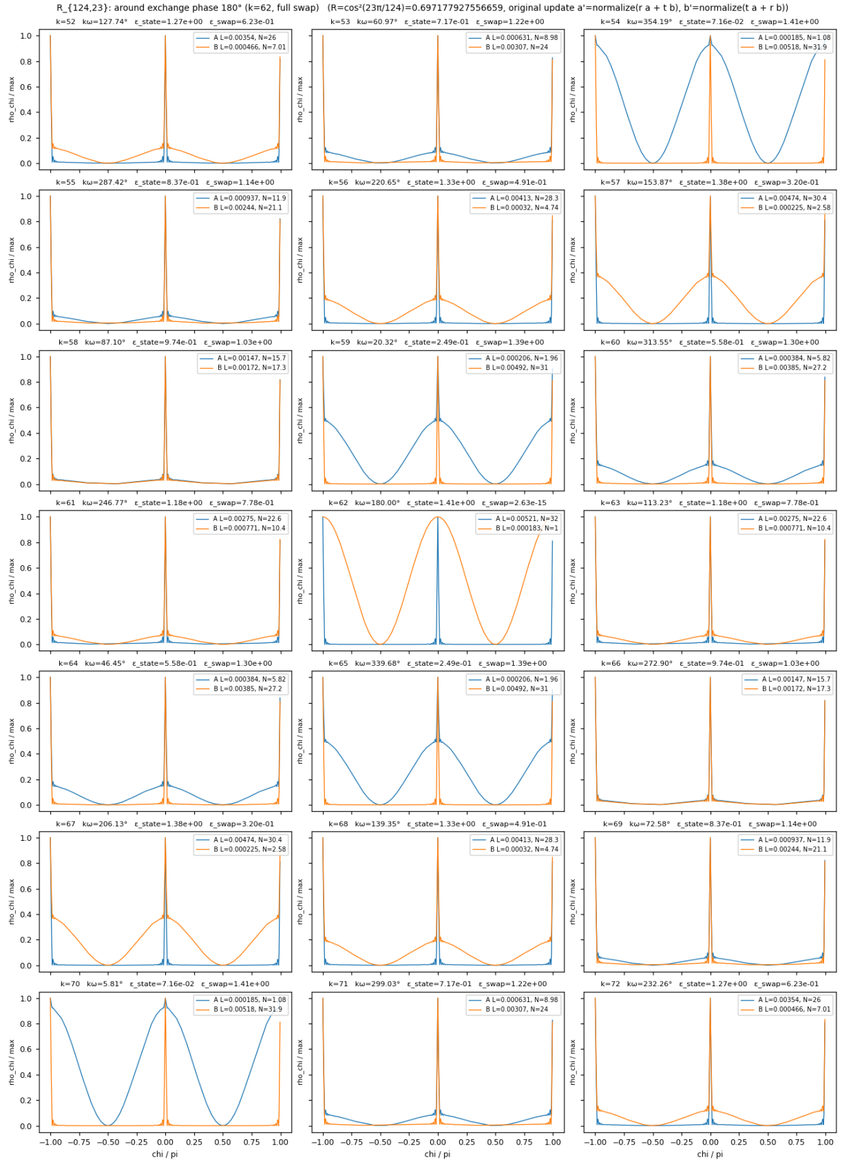
図4 図4：交換位相 180^\circ の前後（衝突 52～72）
