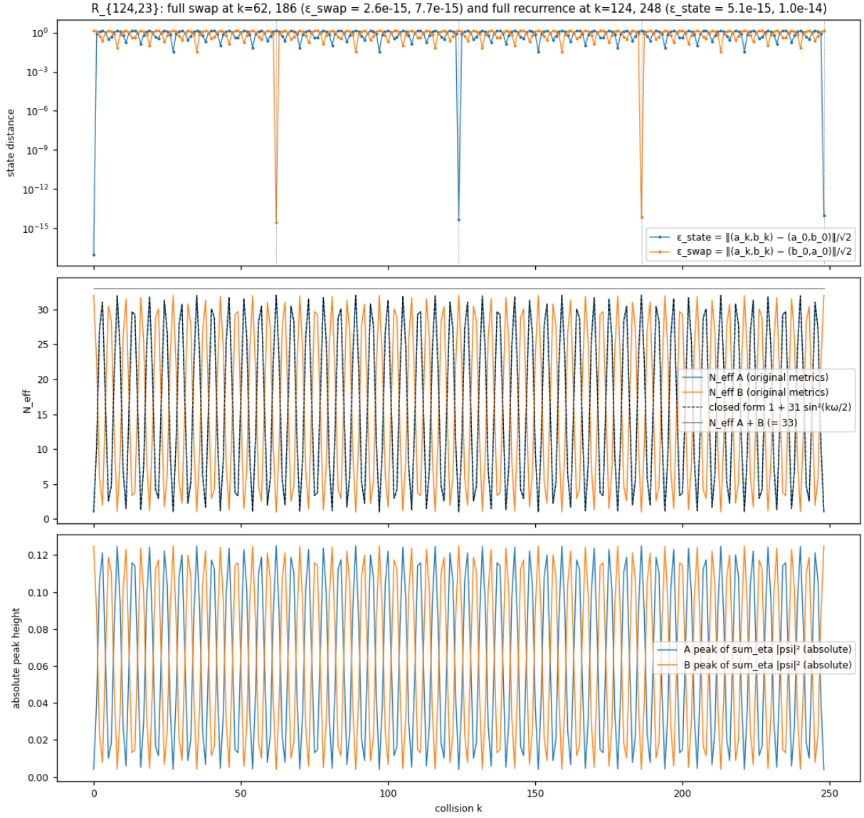
図 6 図 6：厳密根 R_{124,23} における状態距離・有効次数・ピークの絶対高さ（衝突 0～248）
