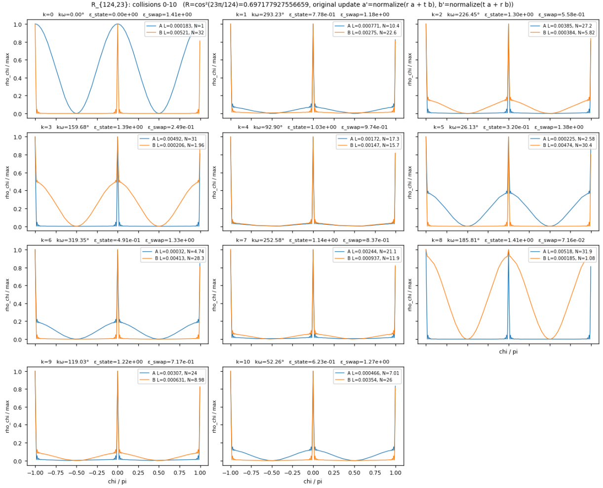
図3 図3: R_{124,23} における二波の波形 (衝突 0~10)
